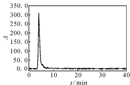
图 1 fac-[ 188 Re(CO) 3 (H 2 O) 3 ] + 的 HPLC 图谱 Fig.1 HPLC of the fac-[ 188 Re(CO) 3 (H 2 O) 3 ] +
